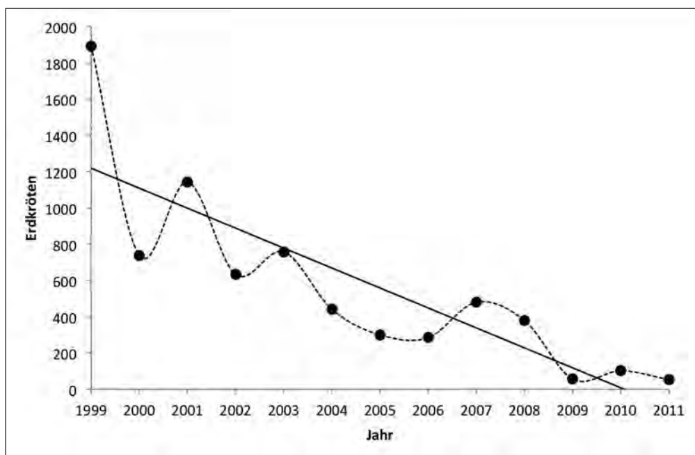
Abb. 3: Beispielhafter negativer Trend registrierter Erdkrötenindividuen an einem Schutzzaun bei Merzig-Weiskirchen (1999-2011). Der (lineare) negative Trend ist statistisch höchst signifikant ( P < 0,001 ); zudem erklärt das lineare Modell 70% Varianz, das Streuungsmaß ist relativ hoch ( CV= 0,91 ).
